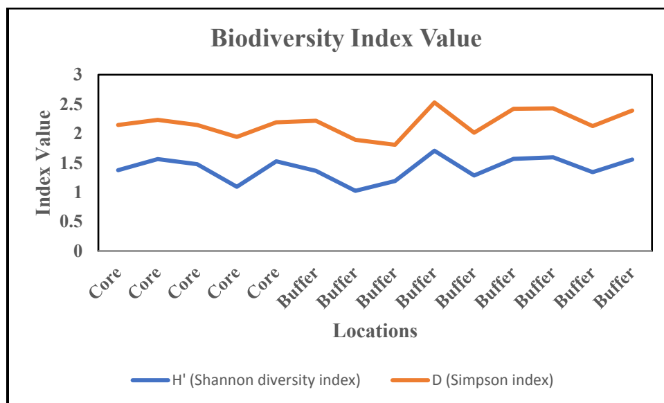
Fig. 3.5. Biodiversity index value
